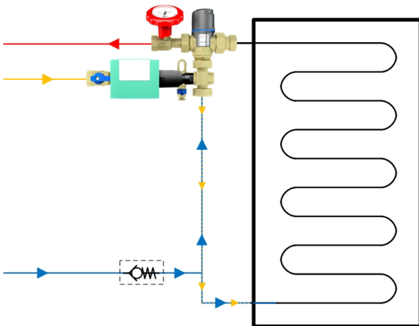
Abbildung 9: Anschluss an einen Hygienespeicher
