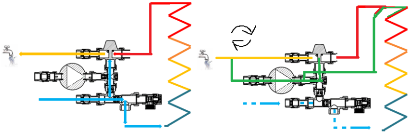
Abbildung 6: (links) Warmwasserentnahme ohne Zirkulation
