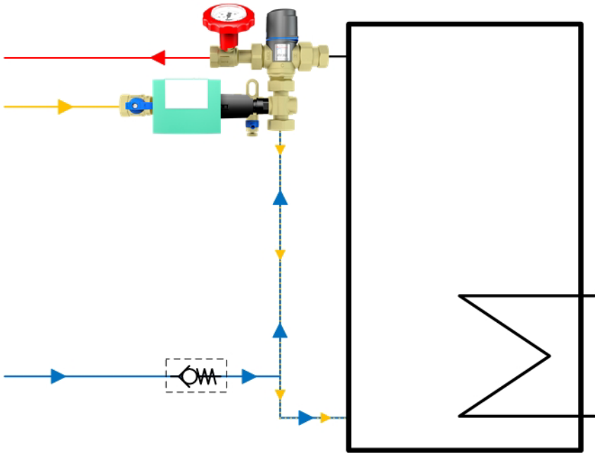
Abbildung 10: Anschluss an einen Trinkwarmwasserbereiter
