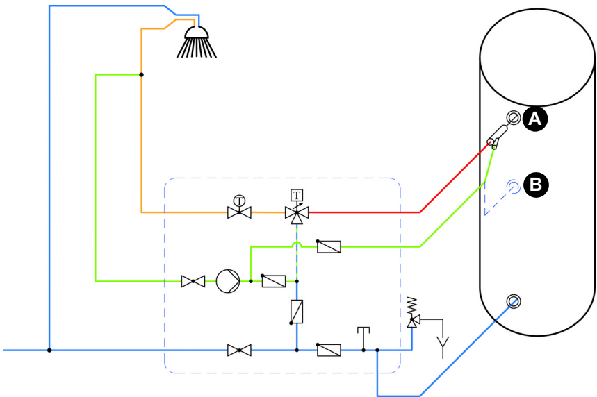
Abbildung 7: (rechts) Warmwasserentnahme während der Zirkulation
