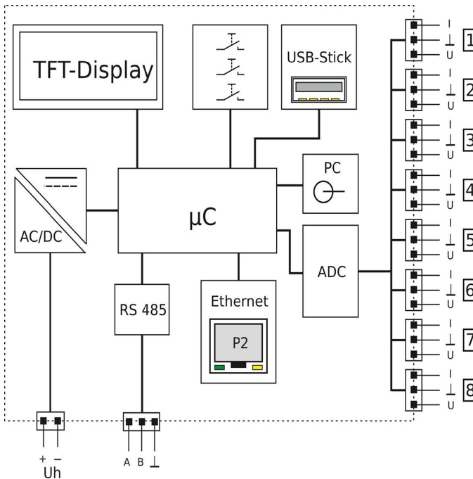
Abbildung 2: Blockschaftbild
