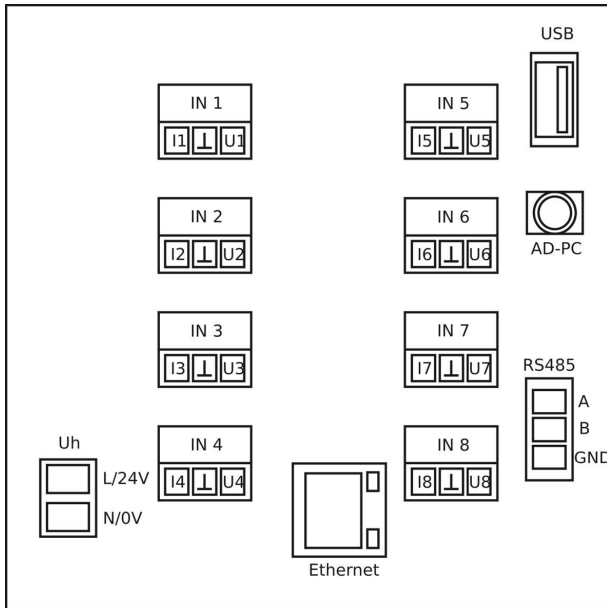
Abbildung 9: Anschlussbelegung Produktrückansicht
